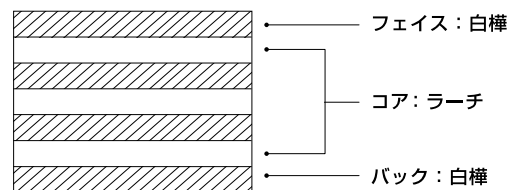
[ 単板構成 ] 7 プライ ( 12 mm )
