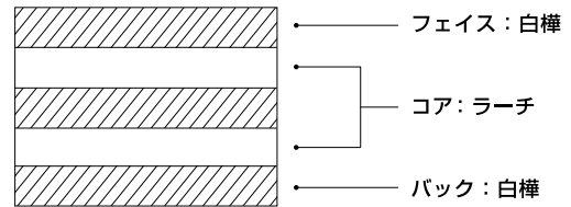
[ 単板構成 ] 5 プライ ( 9.0 mm / 12 mm )
