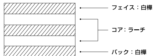
[ 単板構成 ] 5 プライ
