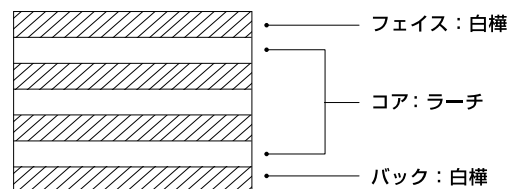
[ 単板構成 ] 7 プライ
